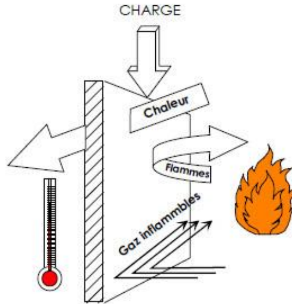
Fig. 15 : CLASSEMENT PARE-FLAMMES
